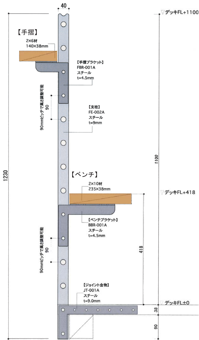
【手摺・ベンチ断面図】
